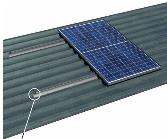
Disposición horizontal de módulos
