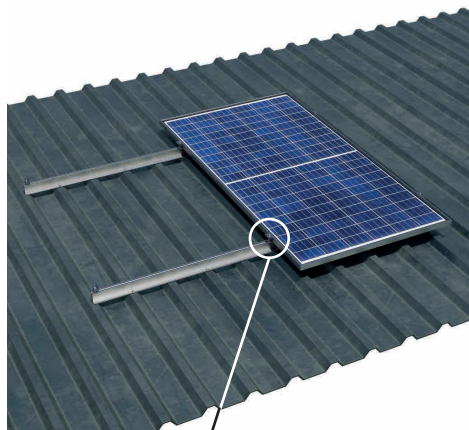
Disposición vertical de módulos
