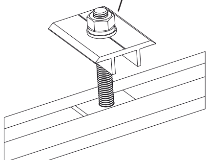
Sistema de fijación intermedia de módulos FV
