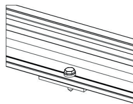
Sistema de fijación a chapa
