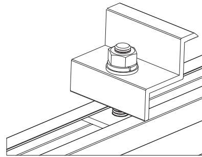
Sistema de fijación final de módulos FV
