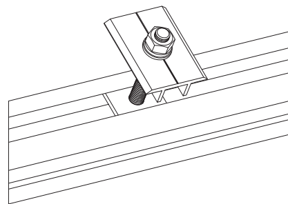
Sistema de fijación intermedia de módulos FV
