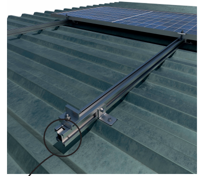
PERFIL R-1000
