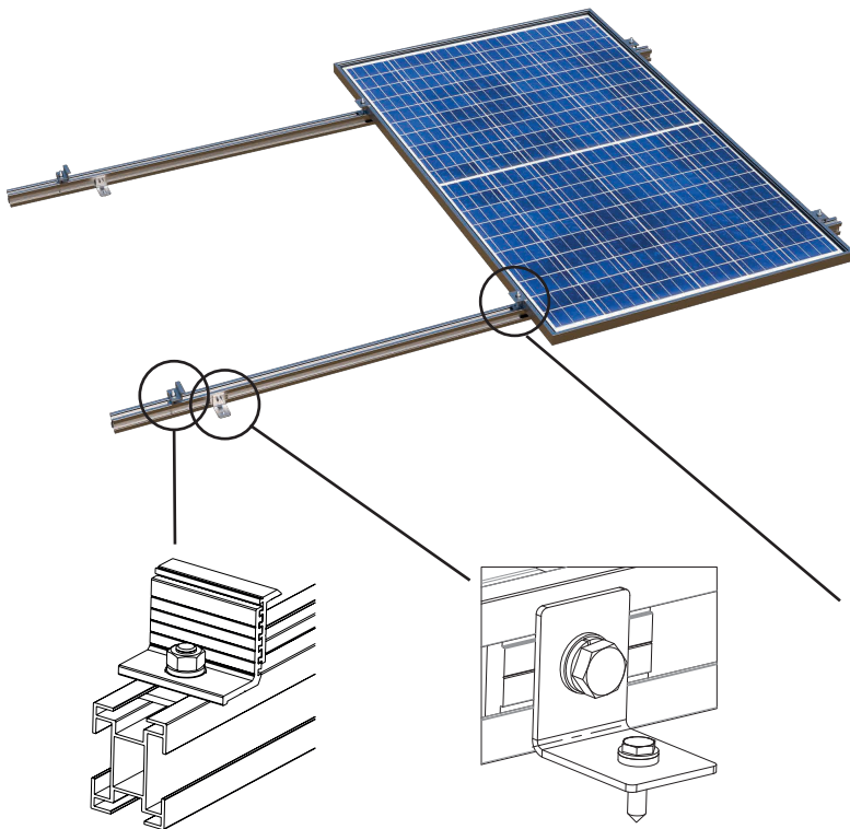
Sistema de fijación final de módulos FV
