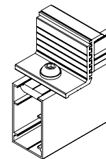
Sistema de fijación final de módulos FV
