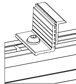
Sistema de fijación final de módulos FV
