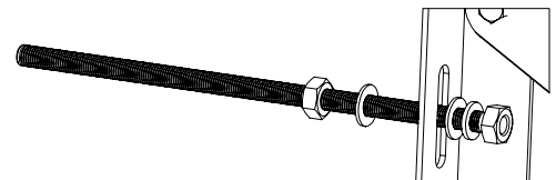
Sistema de anclaje a fachada
