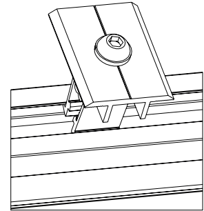
Sistema de fijación intermedia de módulos FV
