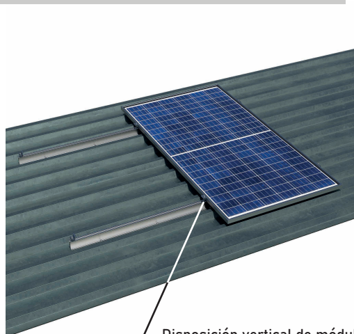
Disposición vertical de módulos
