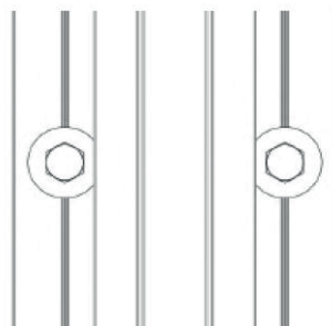
Colación simétrica de tornillos
